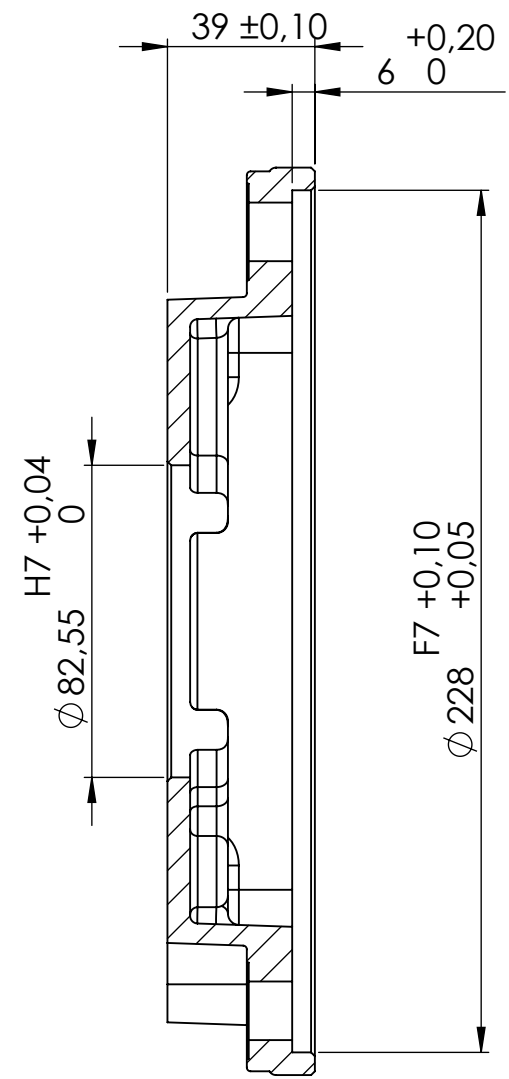
SEZIONE I-I SCALA 1 : 2
