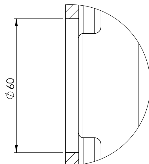
DETTAGLIO H
