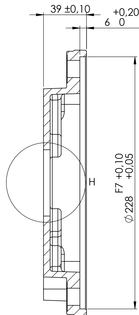
SEZIONE G-G SCALA 1 : 2
