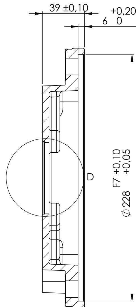
SEZIONE C-C SCALA 1 : 2
