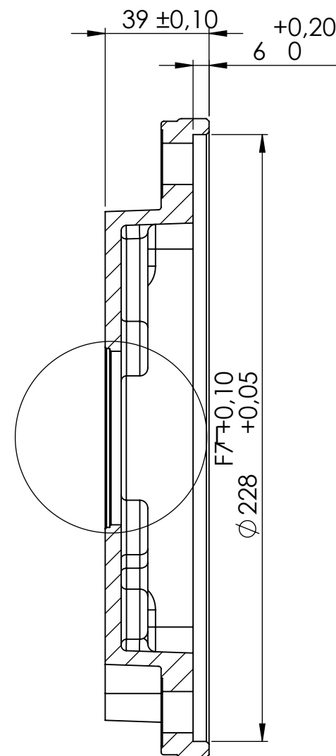
SEZIONE K-K SCALA 1 : 2
