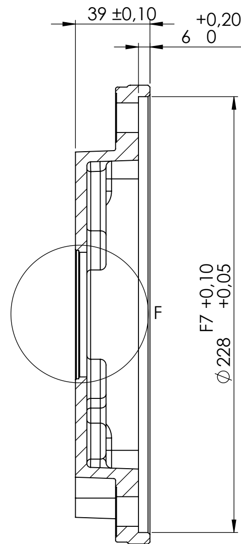
SEZIONE E-E SCALA 1 : 2
