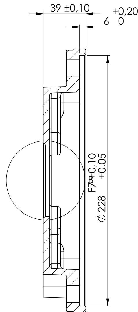
SEZIONE A-A SCALA 1 : 2
